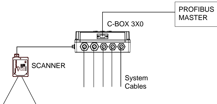
Abbildung 5 – Systemanordnung
