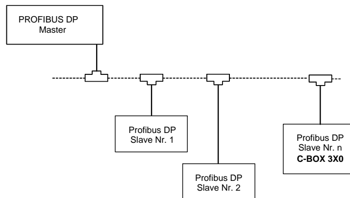
Abbildung 12 - Profibus-Anschluss
